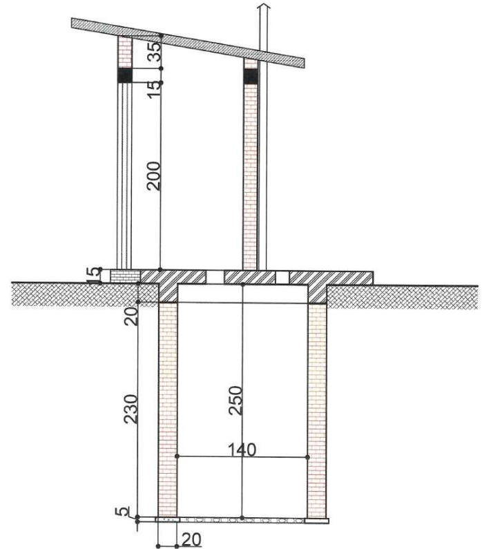
Coupe verticale
