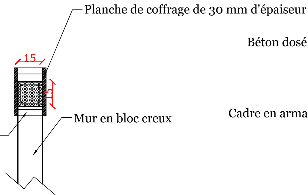
PLAN DE COFFRAGE COLONE
