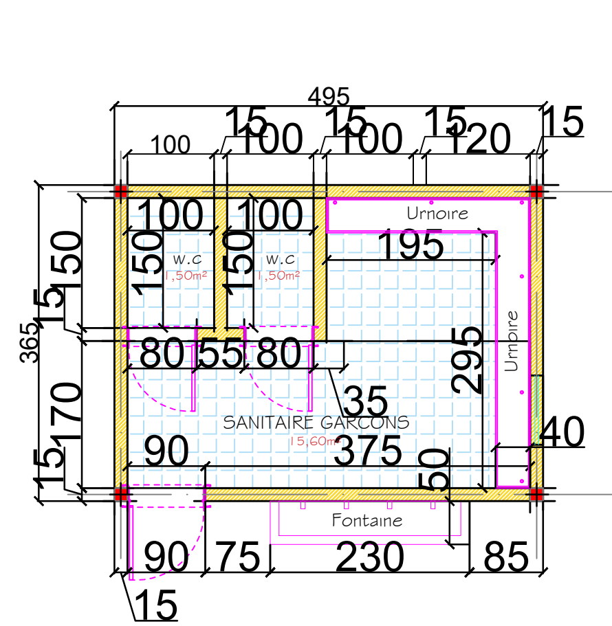
SANITAIRE GARCONS
