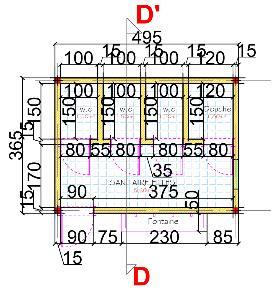
SANITAIRE FILLES
