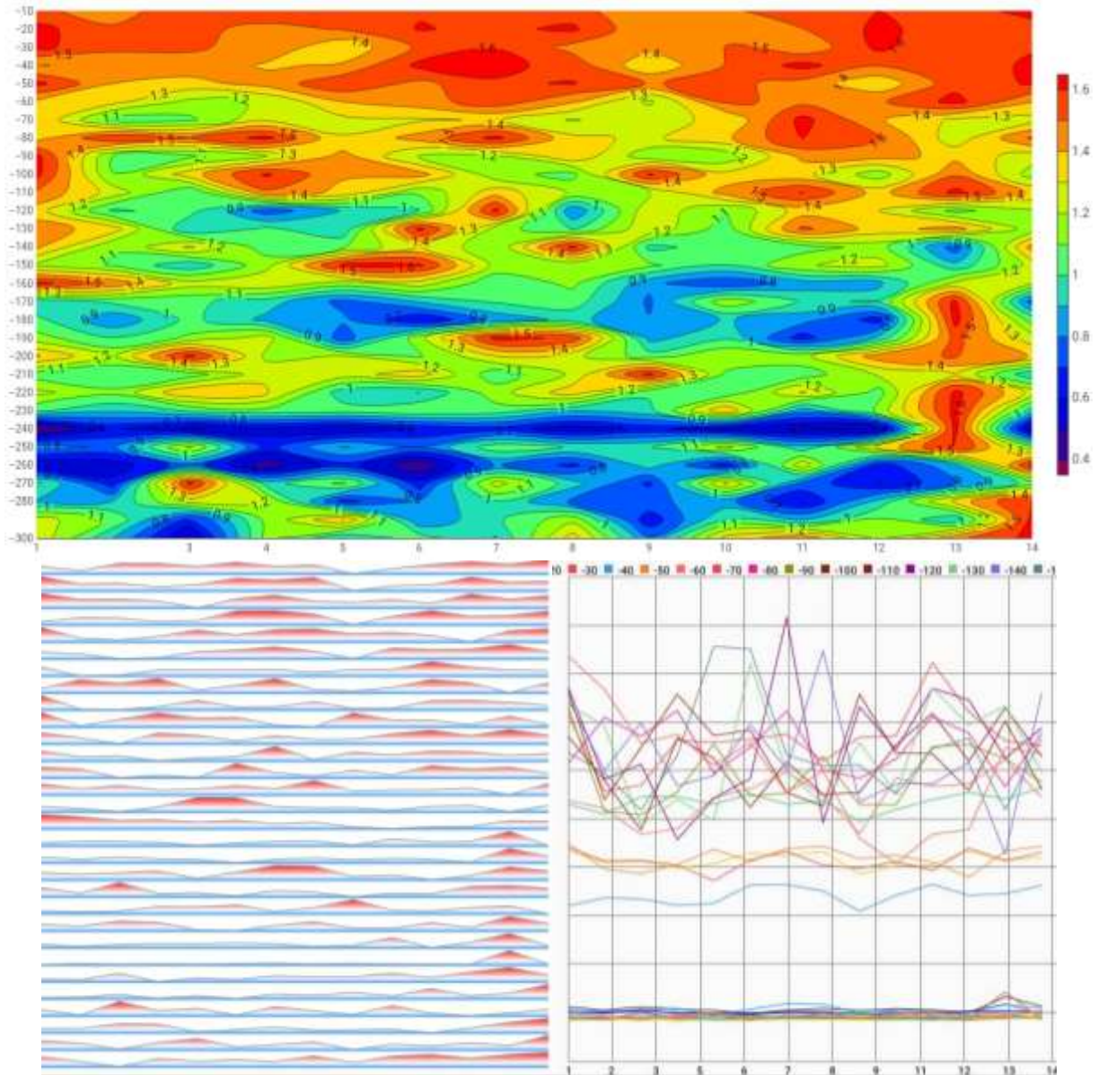
Figure 1: coupe géo électrique et diagrammes d'anomalie de l'Ep 2 Kamilabi
