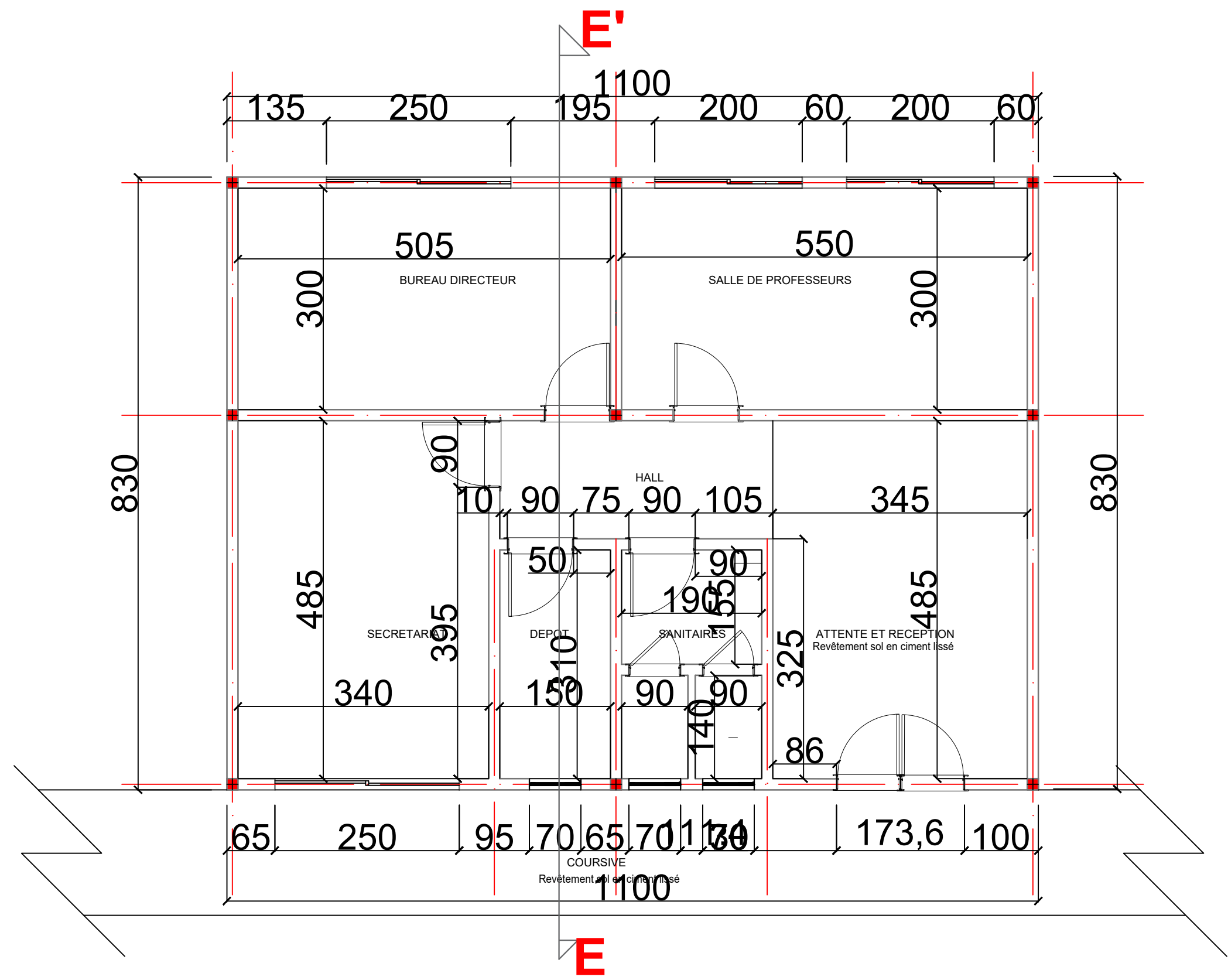
VUE EN PLAN COTEE BLOC ADMINISTRATION
