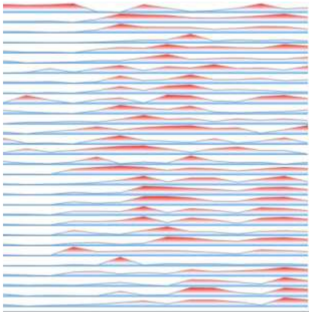
Coupe géo électrique et diagrammes d'anomalie
