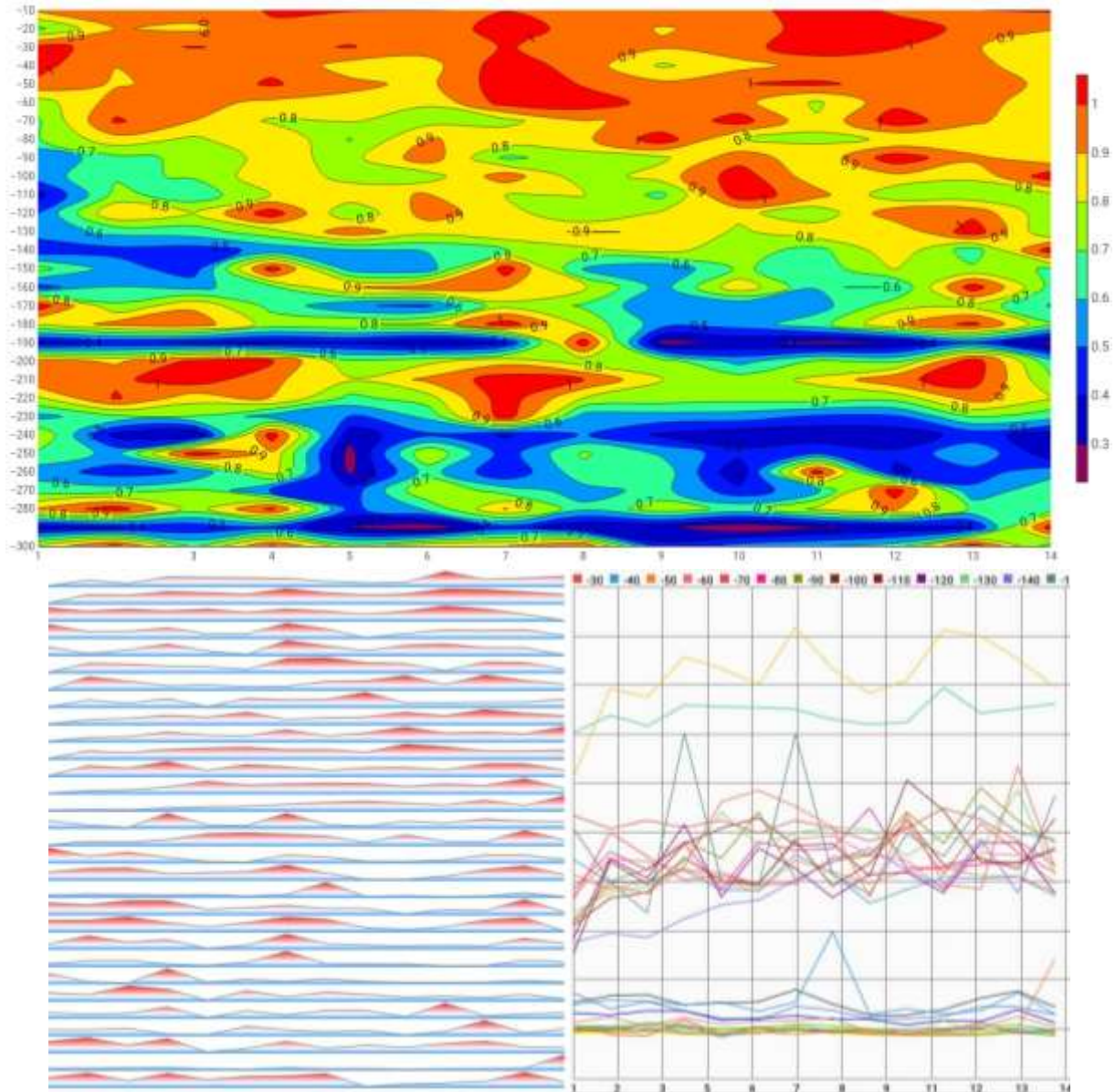
Figure 1: coupe géo électrique et diagrammes d'anomalie de l'Ep Tshisubulu
