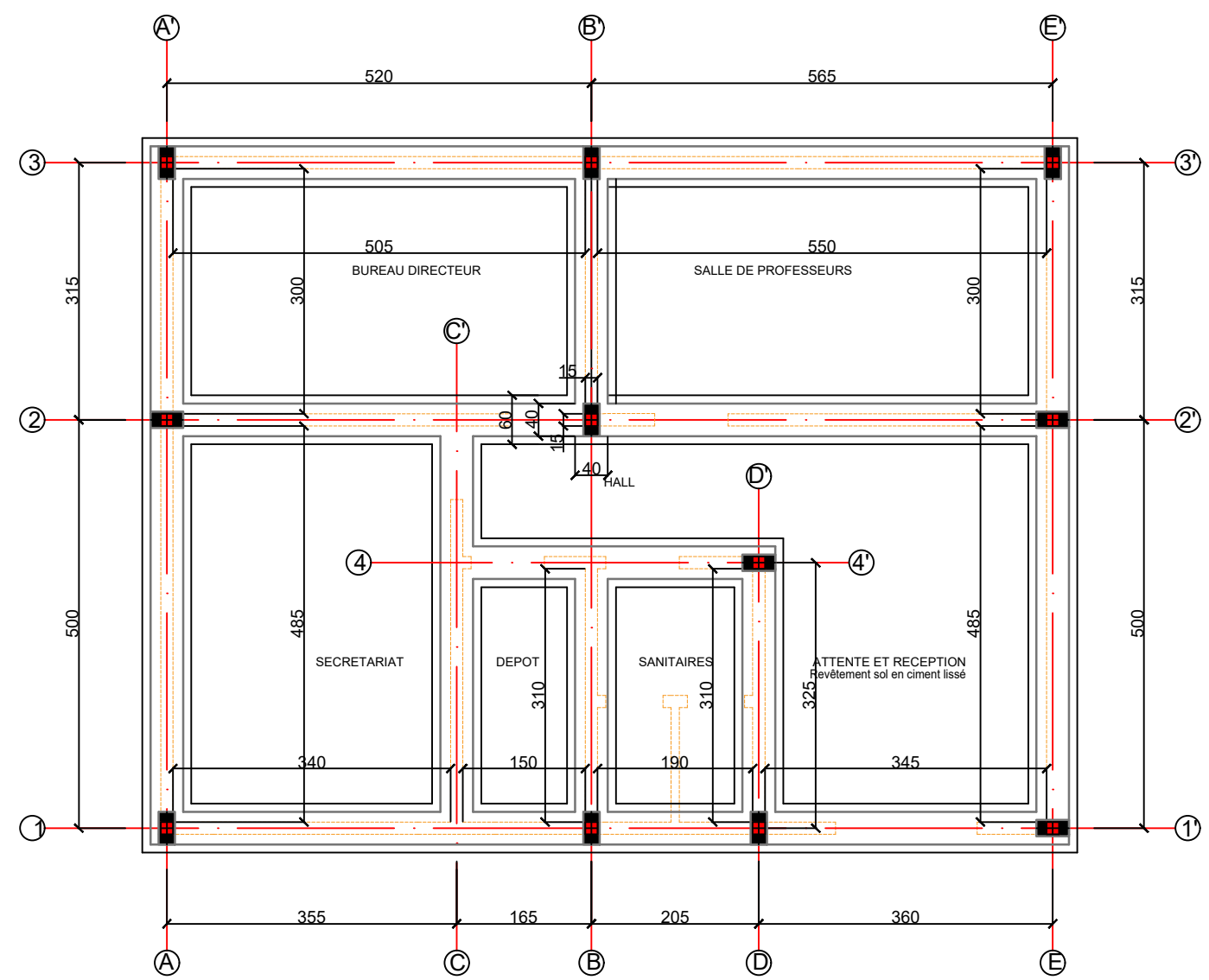
PLAN DE FONDATION BLOC ADMINISTRATION
