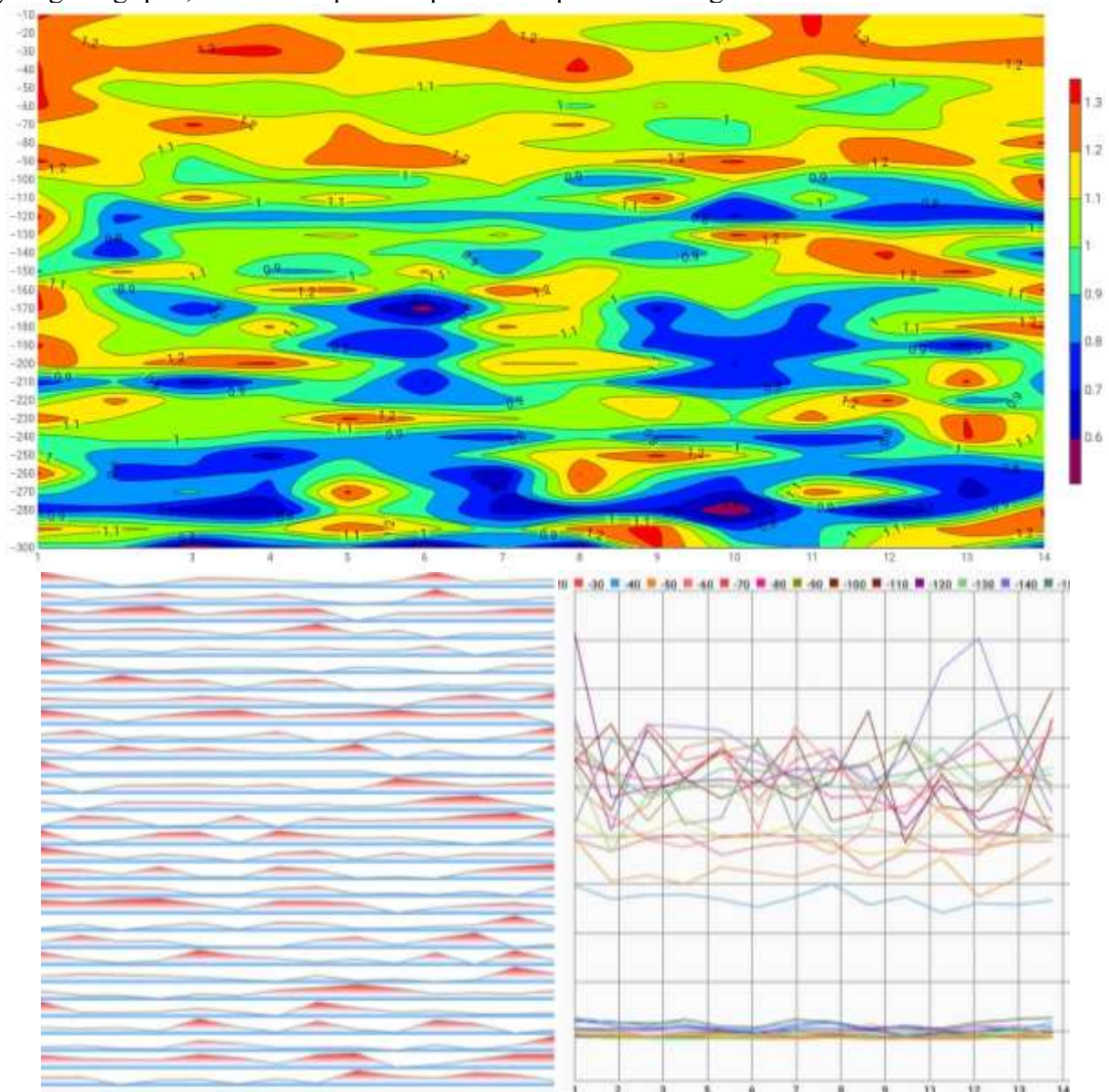
Figure 1 : coupe géo électrique et diagrammes d'anomalie de l'Ep Ipanga
