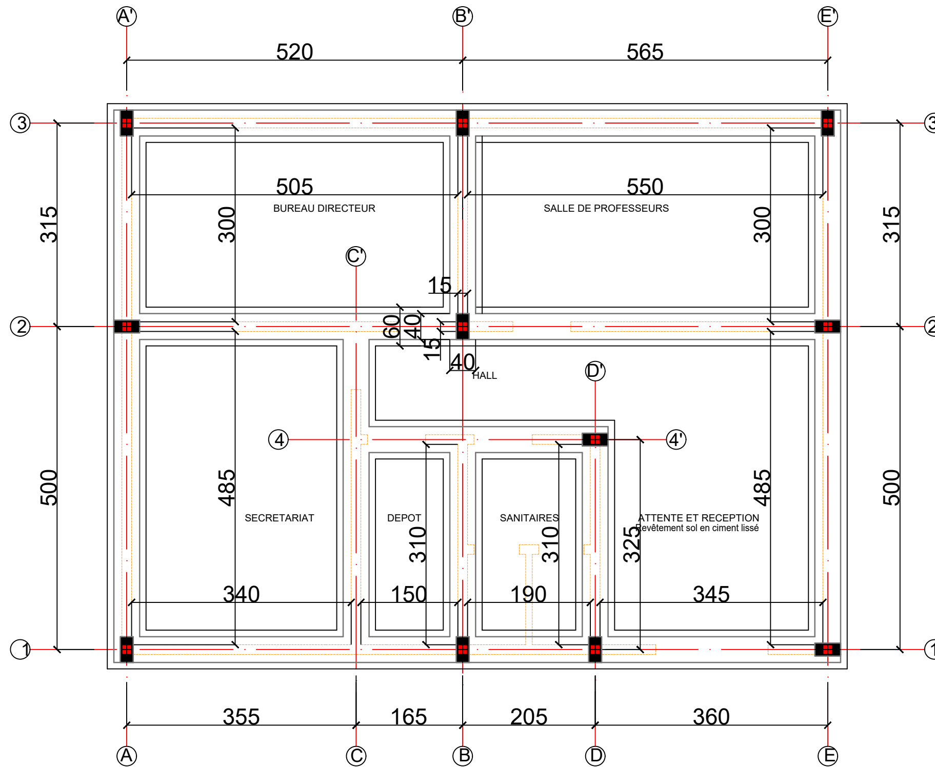
PLAN DE FONDATION BLOC ADMINISTRATION
