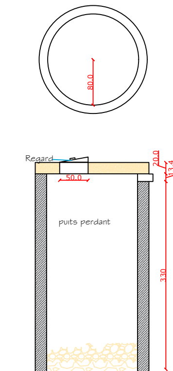
PUIT PERDANT
