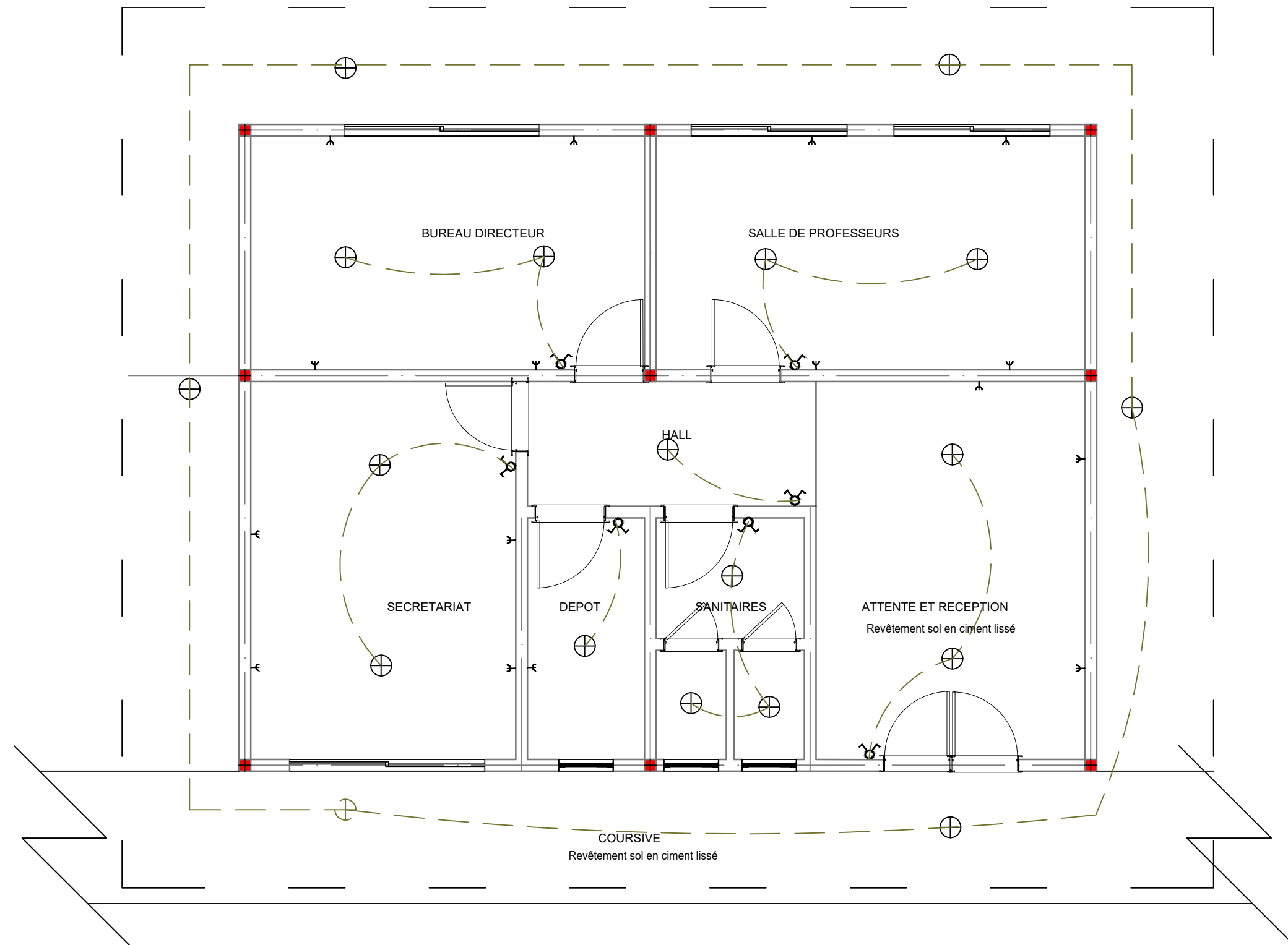
PLAN D'ELECTRICITE BLOC ADMINISTRATION
