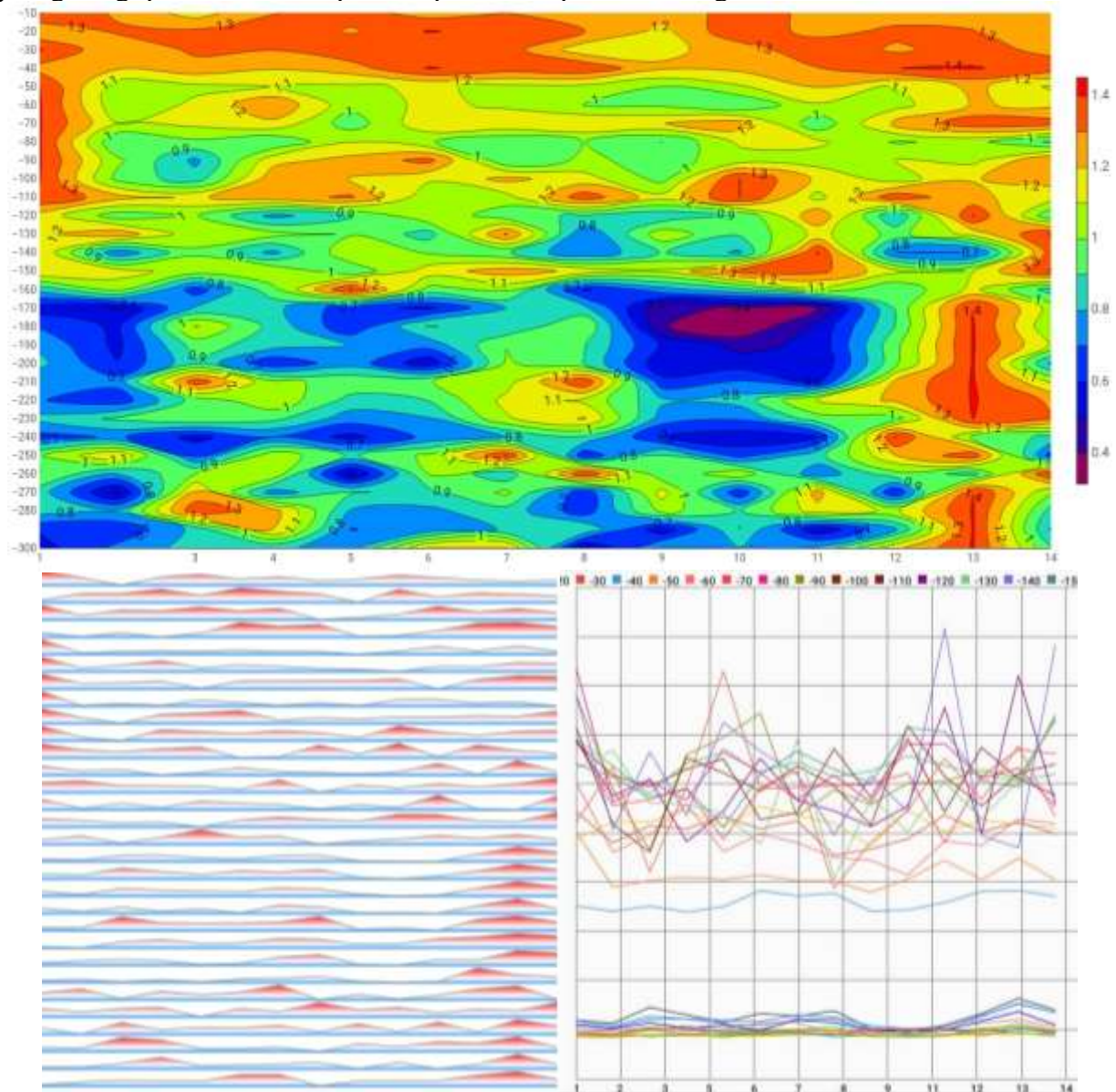
Figure 1: coupe géo électrique et diagrammes d'anomalie de l'Ep Saint Aimerance
