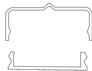
PROFILE LATERAL ALUMINIUM AVEC CLIPS
