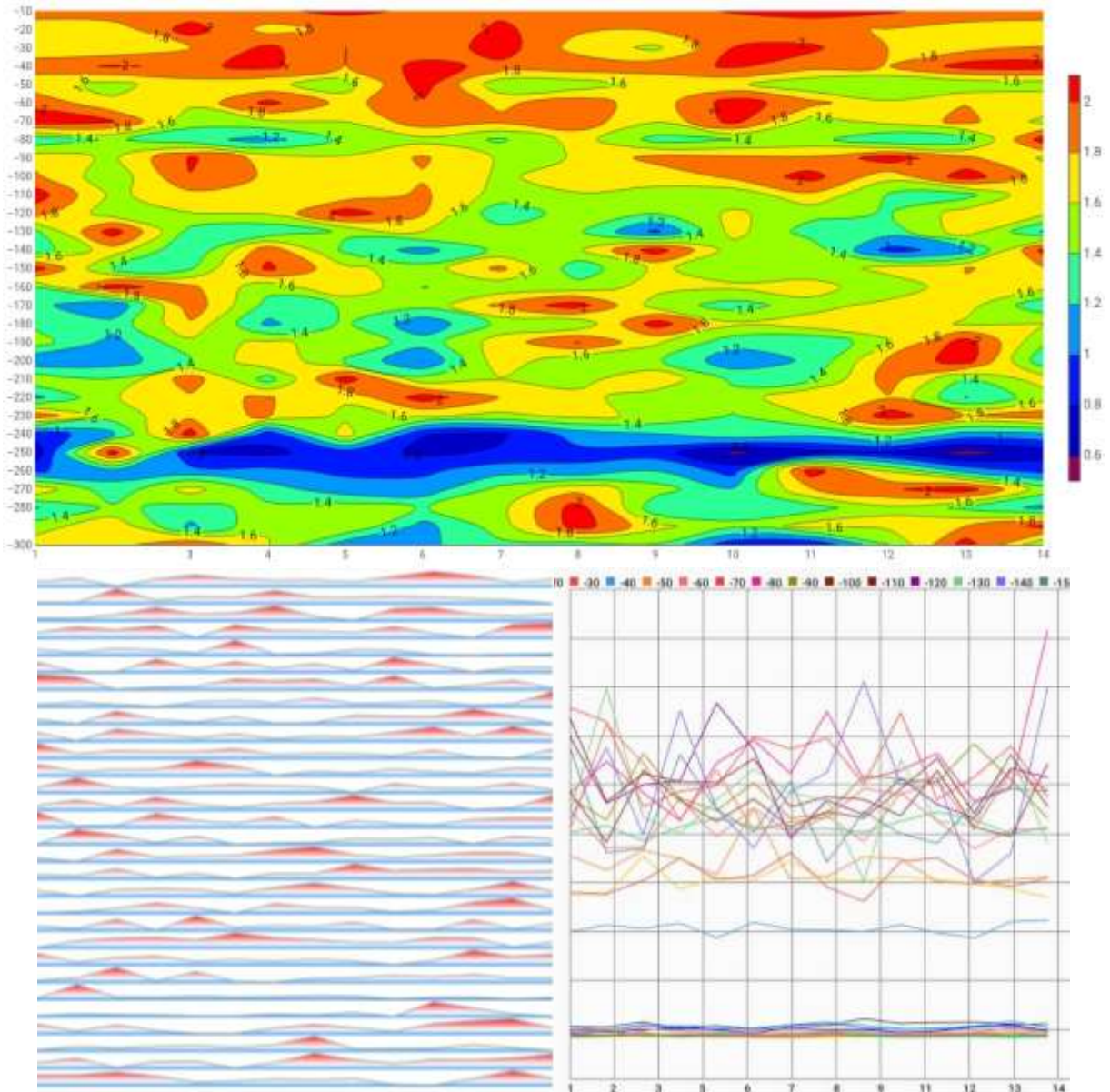
Figure 1: coupe géo électrique et diagrammes d'anomalie de l'Ep Lubumba
