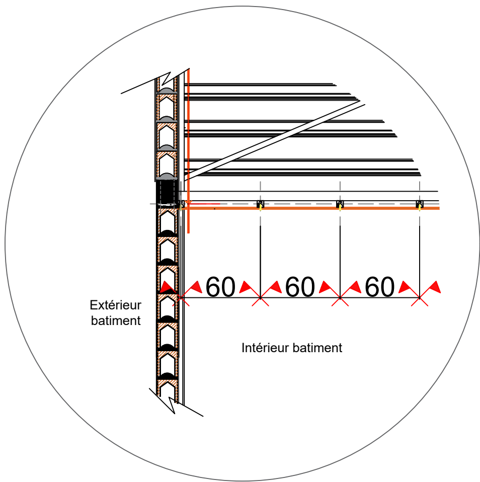
Détail Toiture
