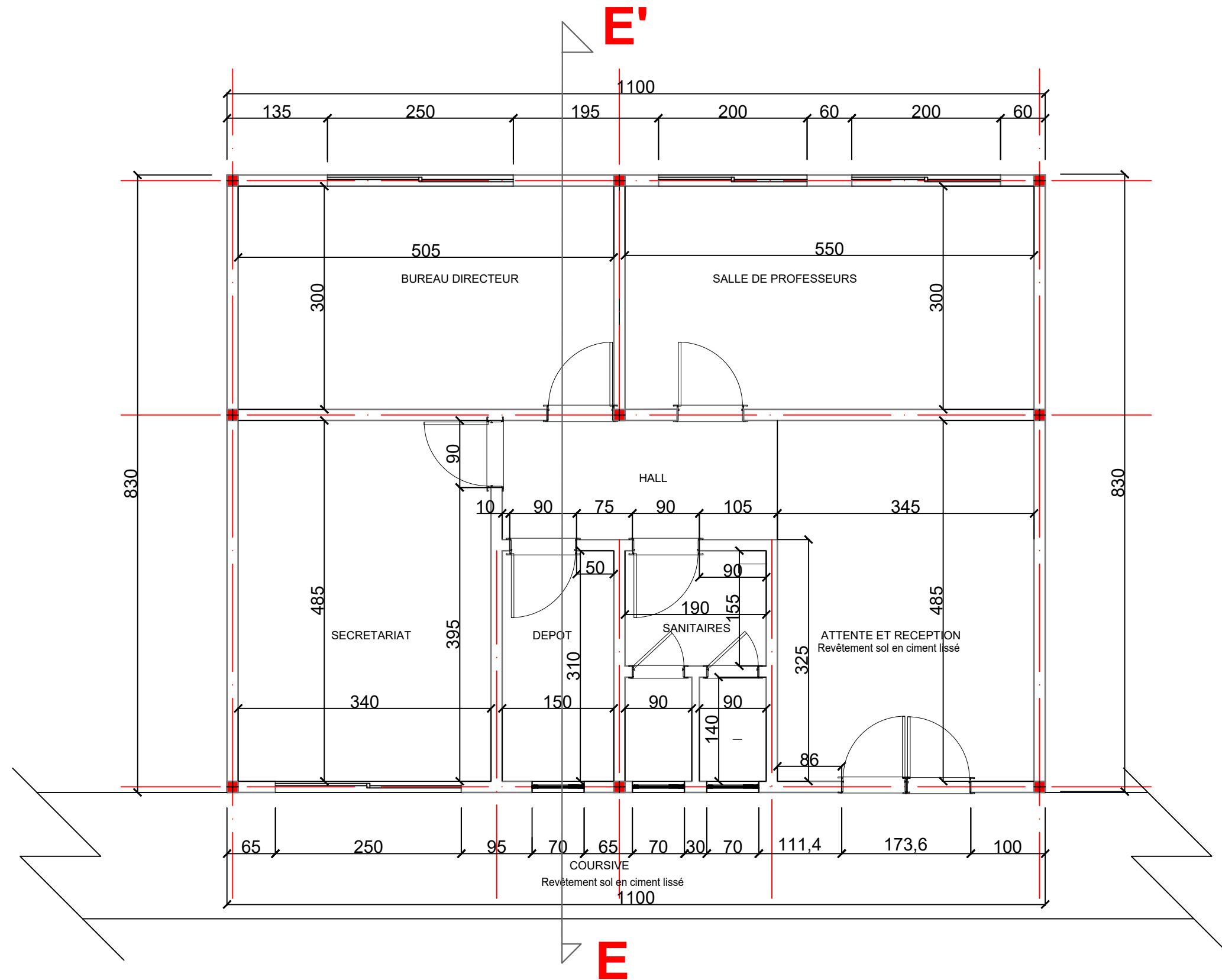
VUE EN PLAN COTÉE BLOC ADMINISTRATION
