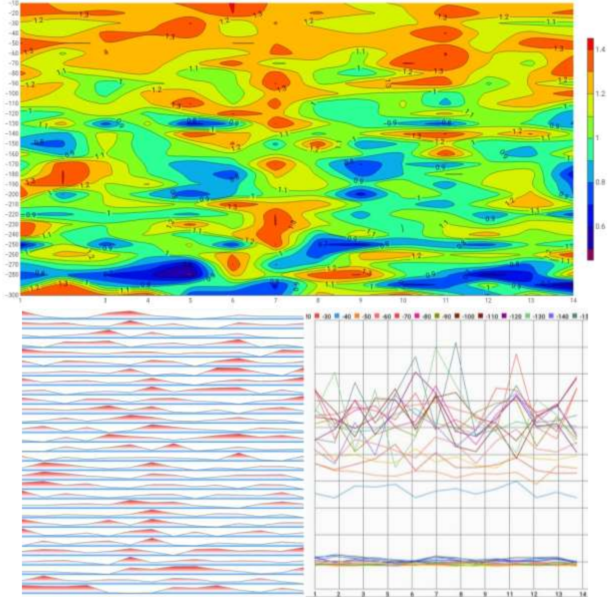
Figure 1: coupe géo électrique et diagrammes d'anomalie de l'Ep Tatalayi
