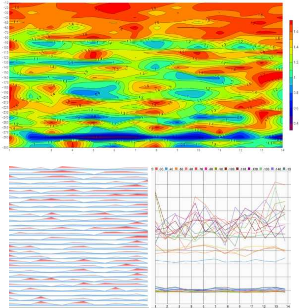
Figure 3 : diagramme processus et des zones d'anomalies de l'Ep Mudukulu
