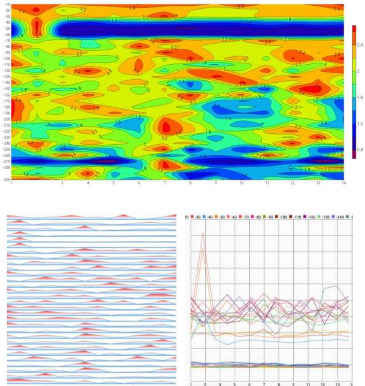
Figure 1 : diagramme processus et des zones d'anomalies de Ep 2 Dikolelayi
