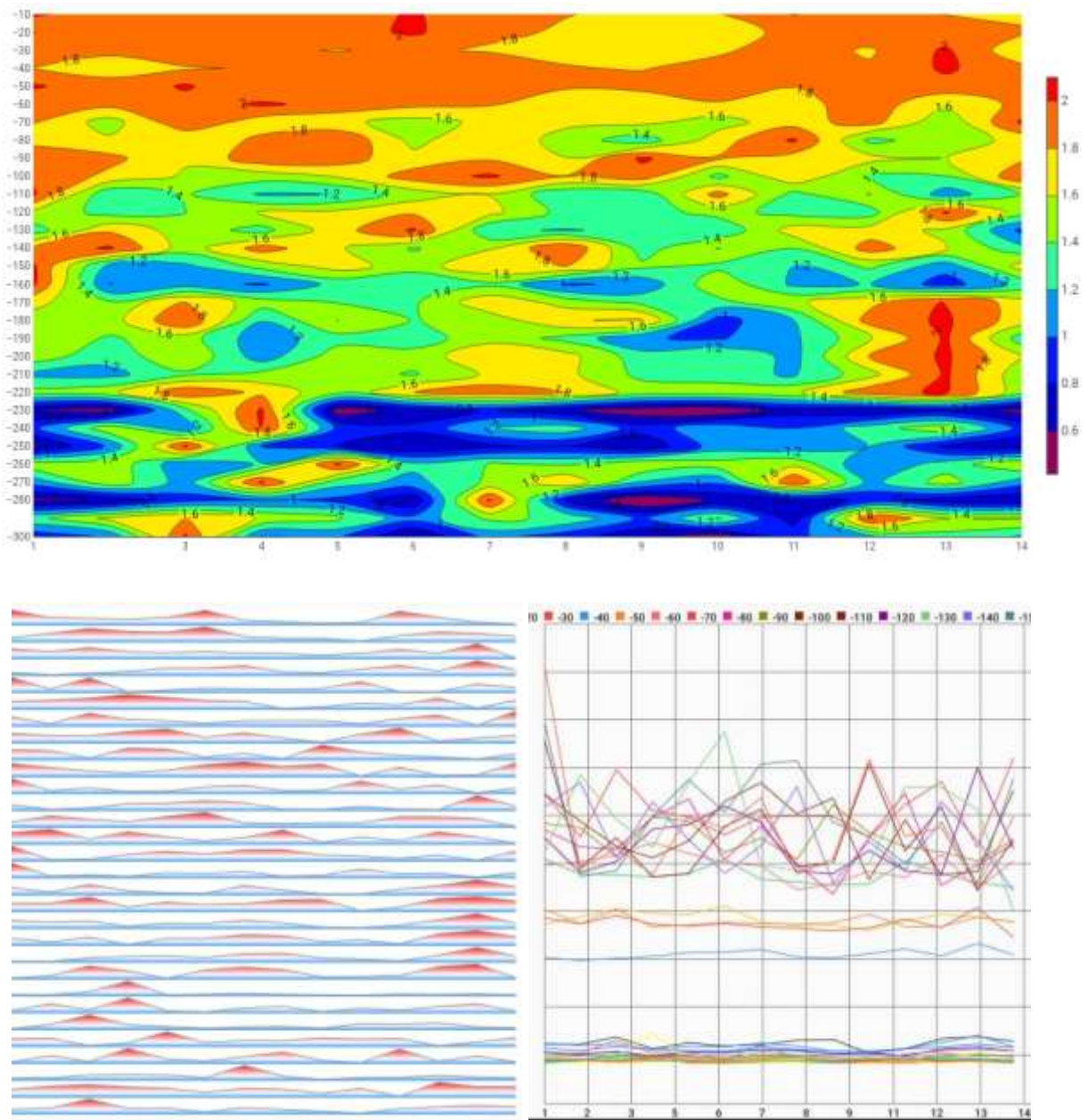
Figure 2 : diagramme processus et des zones d'anomalies de l'Ep 3 Kamayi
