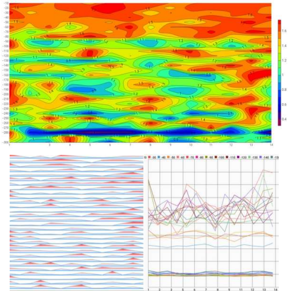
Figure 4: coupe géo électrique et diagrammes d'anomalie de l'Ep Nsanga nyembue
