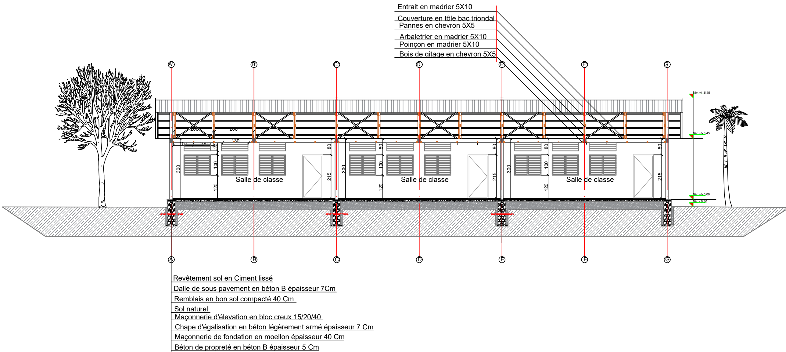
COUPE B-B' BLOC SALLE DE CLASSE
