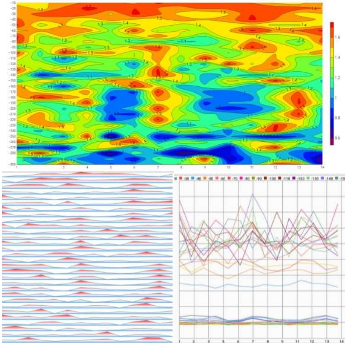
Figure 1 : coupe géo électrique et diagrammes d'anomalie de l'Ep Bakua tshibusu
