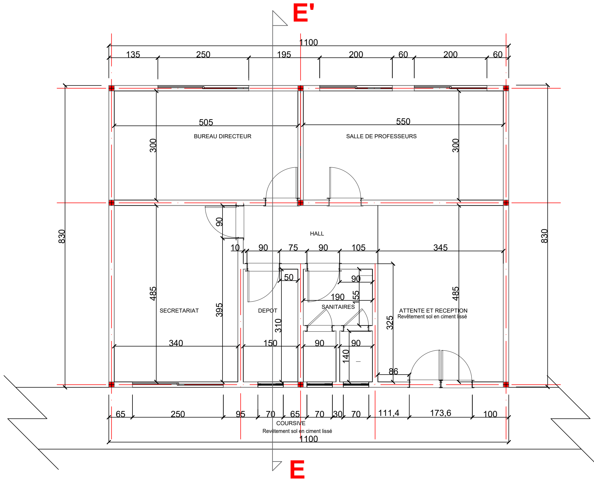
VUE EN PLAN COTEE BLOC ADMINISTRATION
