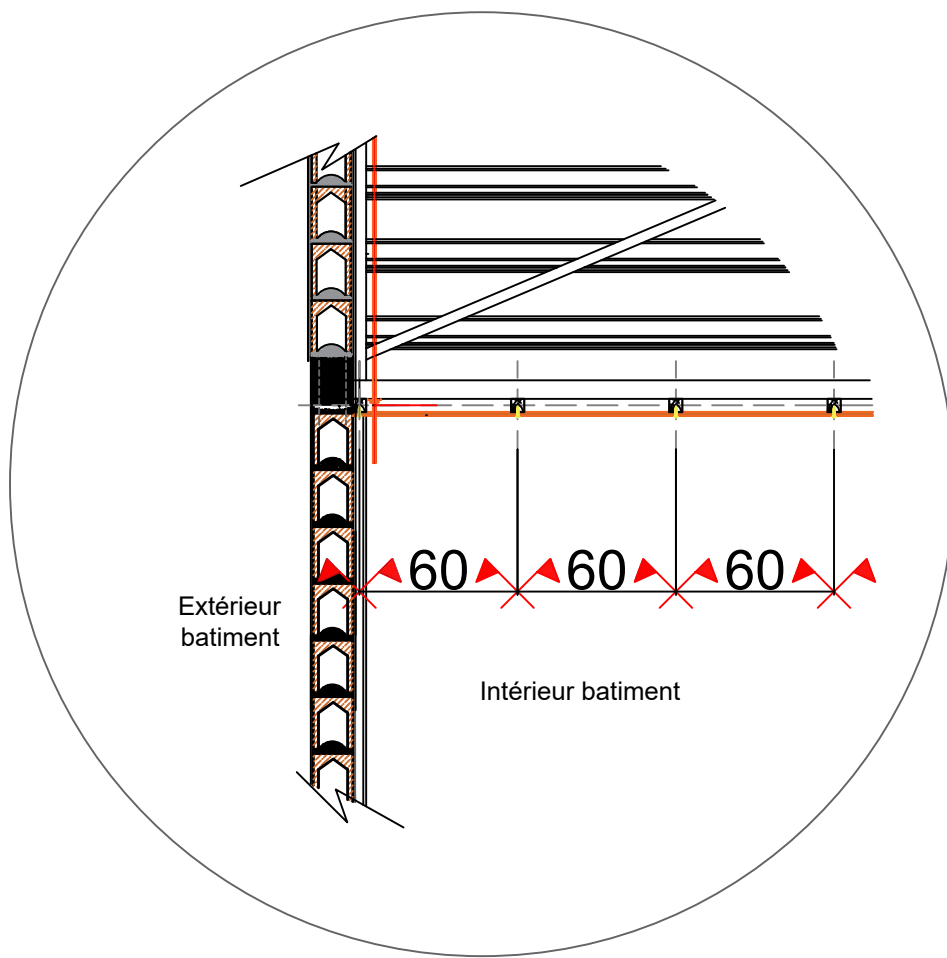
Détail Toiture
