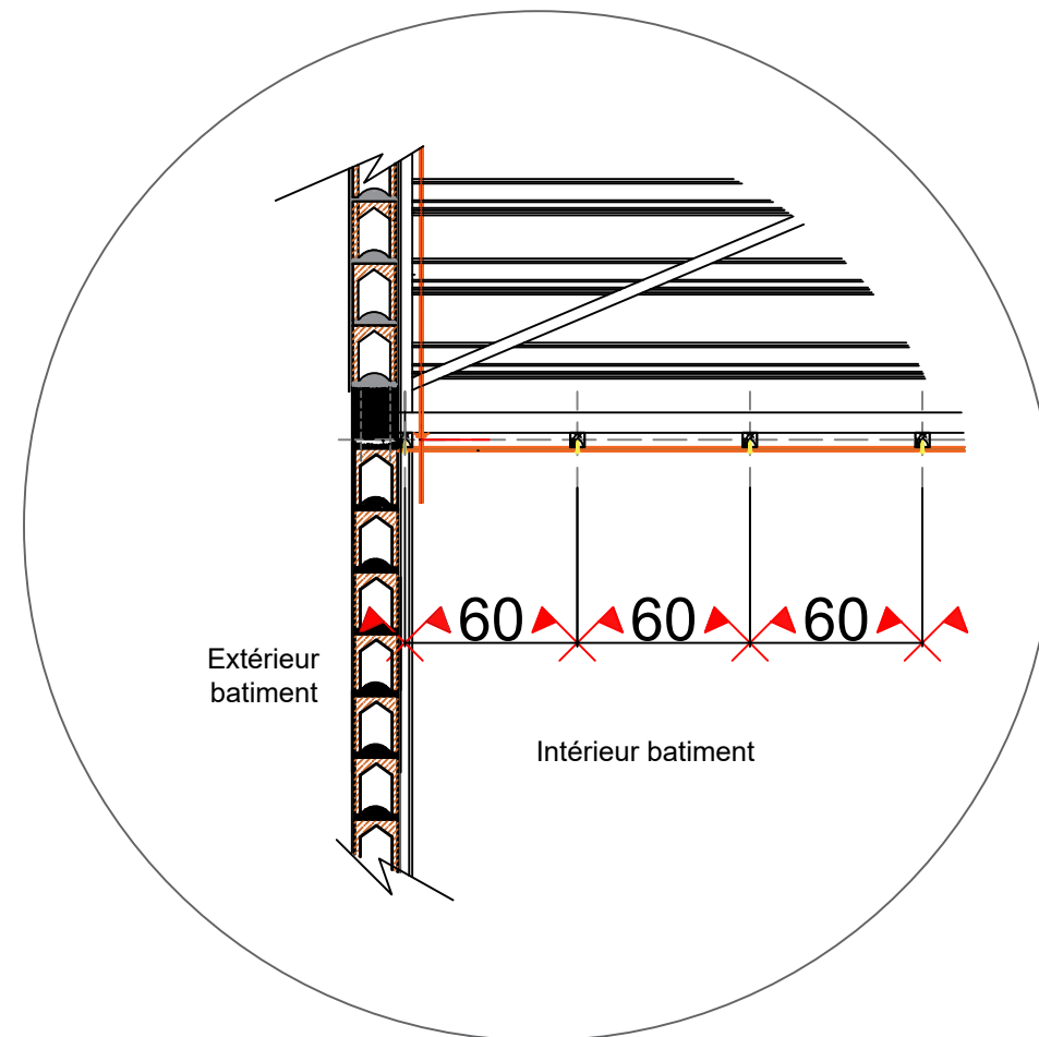
Détail Toiture
