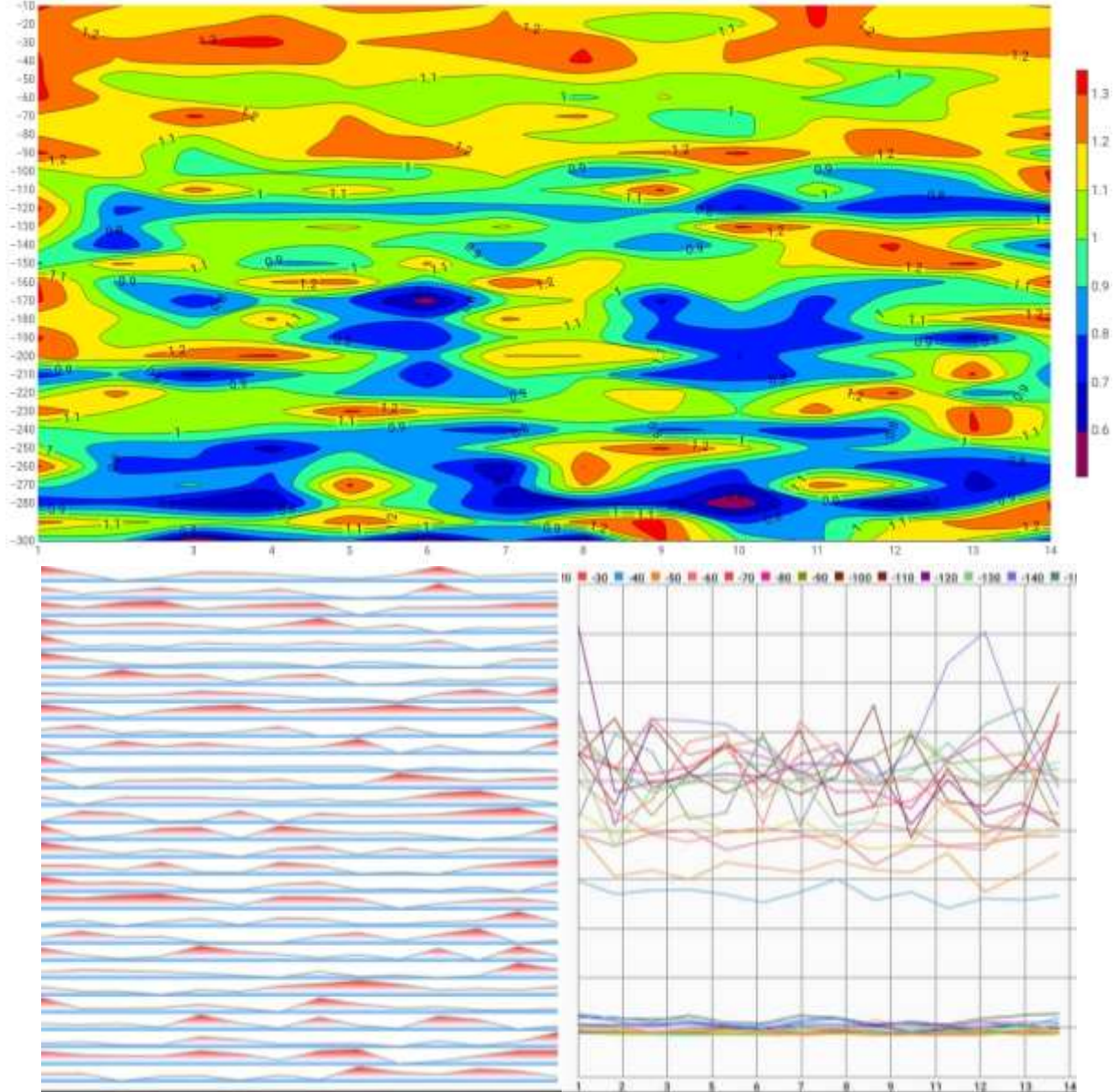
Figure 1: coupe géo électrique et diagrammes d'anomalie
