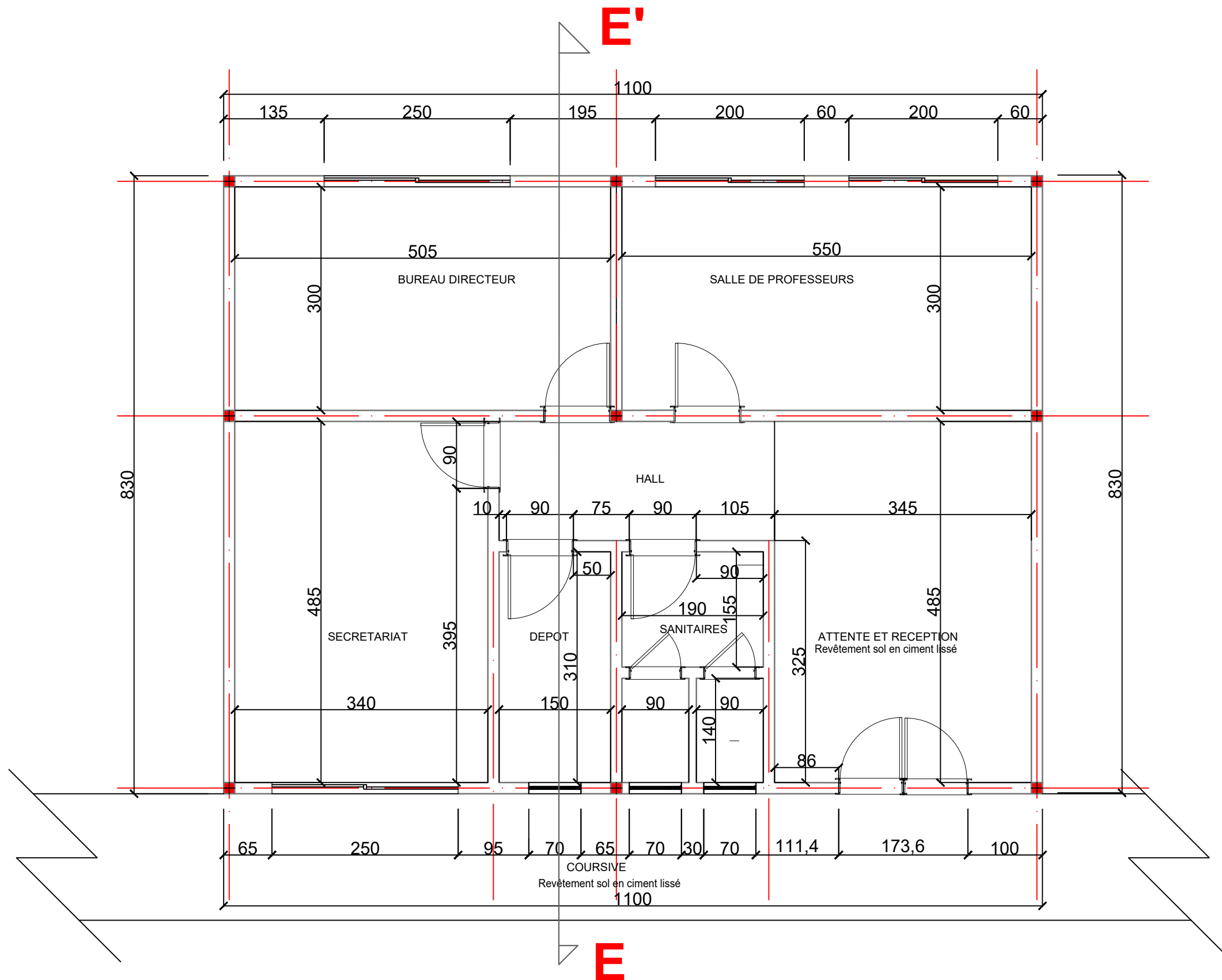
VUE EN PLAN COTÉE BLOC ADMINISTRATION
