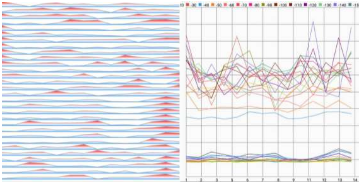
Figure 1: coupe géo électrique et diagrammes d'anomalie de l'Ep Mukengela
